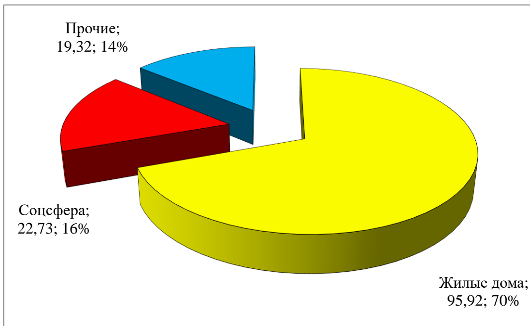
Тепловые нагрузки по объектам значимости от котельных ООО «ОК и ТС», г. Котлас
